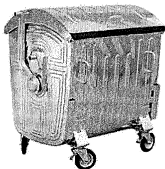
Рисунок – 24 Евроконтейнер оцинкованный вместимостью 1,1 м 3
